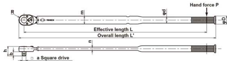
BQSP400N
